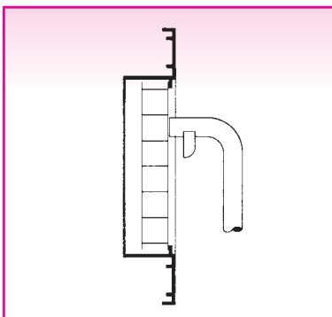
Vélocimètre avec sonde: 2220 A ou 6070
